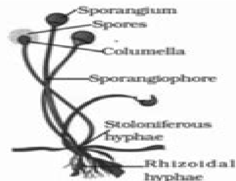
Fig. 2.4 Rhizopus
